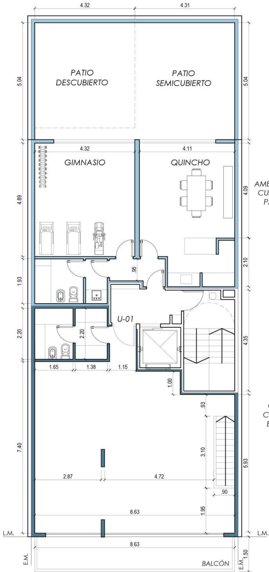
1° PISO esc 1:100
