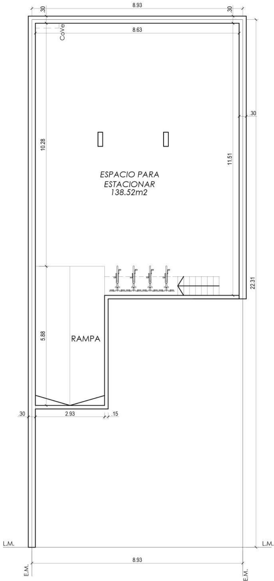
subsuelo esc 1:100
